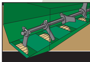
SEED BOX AGITATOR
